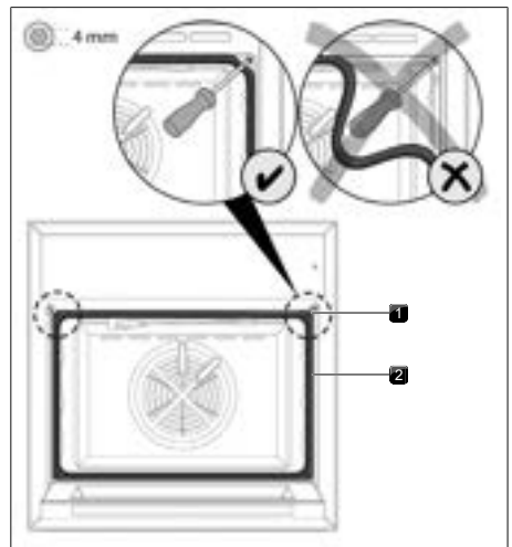
Rys. 8.16 Mocowanie urządzenia
