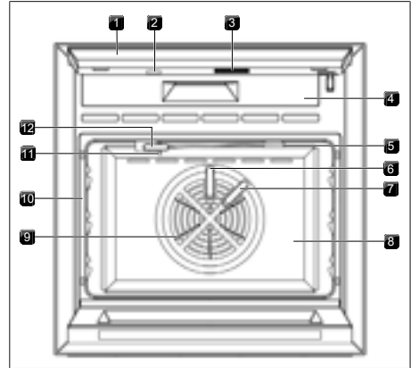
Rys. 4.1 Budowa, część 1
