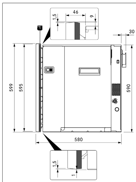
Rys. 8.2 Wymiary urządzenia
